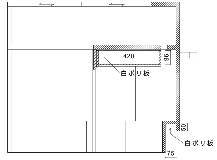
A-A' 断面
